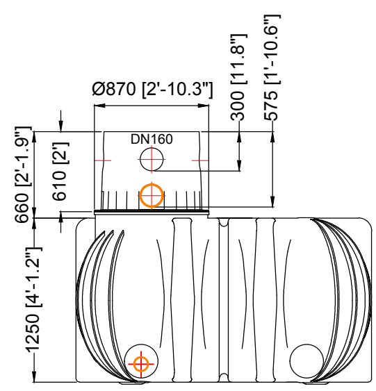
Ansicht A / view A
